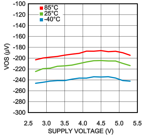
Input V OS_RW vs. VDD (V bias 0mV)
